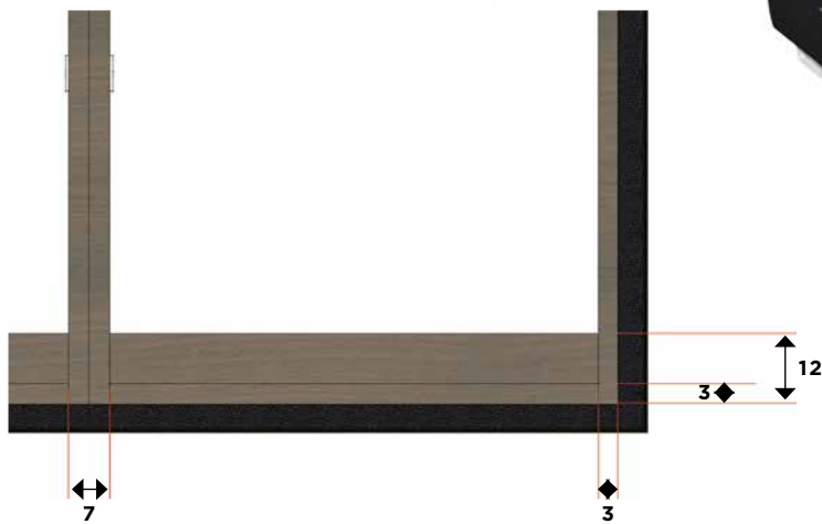
Draufsicht Detailausschnitt Fußteil:
