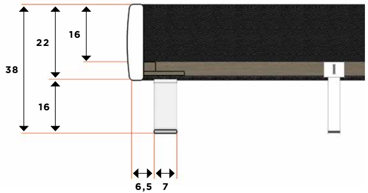
Seitenansicht Detailausschnitt Fußteil:
