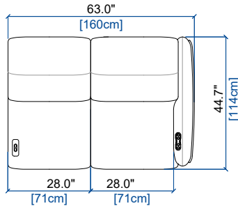
152 BATARD 1.5 PL. ACC. DROIT (EN 2 PARTIES) - FULL RELAX 1.5-SEAT 1-ARM UNIT RIGHT ARM. (IN 2 PARTS) - FULL RELAX BATARD 1.5 PL. APOY. DER. (EN 2 PARTES) - FULL RELAX
