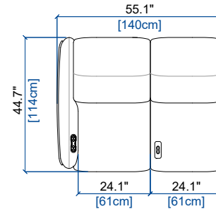
51P PETIT BATARD 1.5 PL. ACC. GAUCHE (EN 2 PARTIES) - FULL RELAX SMALL 1.5-SEAT 1-ARM UNIT LEFT ARM. (IN 2 PARTS) - FULL RELAX BATARD 1.5 PL. APOY. IZQ. PEQ. (EN 2 PARTES) - FULL RELAX
