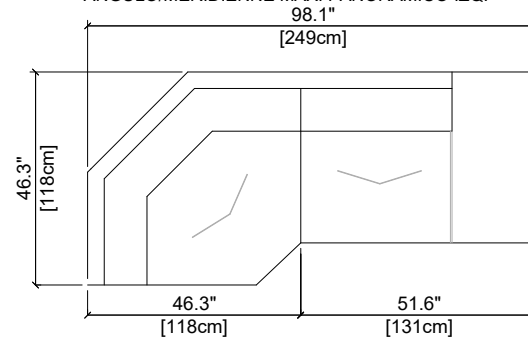
8M ANGLE/MERIDIENNE MAXI PANORAMIQUE GAUCHE MAXI PANORAMIC CORNER/MERIDIENNE LEFT ANGULO/MERIDIENNE MAXI PANORAMICO IZQ.
