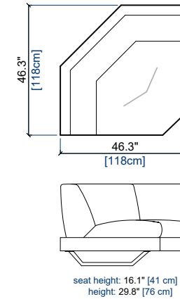
230 ANGLE PANORAMIQUE DROIT ACC. GAUCHE RIGHT PANORAMIC CORNER ELEMENT, LEFT ARM ANGULO PANORAMICO DERECHO APOY. IZQU.
