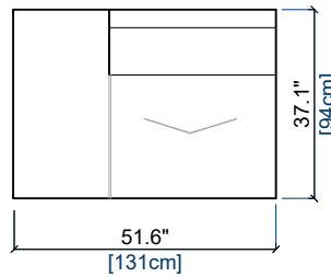
226 MOYEN TERMINAL GAUCHE INDEP. MEDIUM END UNIT LEFT INDEP. MEDIANA TERMINAL IZQUIERDO INDEP.
