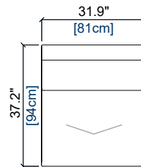
S1S CHAUFFEUSE INDEP. - GAUCHE INDEP. ARMLESS CHAIR - LEFT CHAUFFEUSE INDEP. - IZQ.
