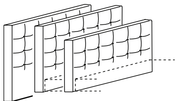
BOHEMIAN C schwebend / hovering Höhe / height: 94/114cm BOHEMIAN C aufstehend / standing Höhe / height: 136cm Tiefe / depth: 10cm Breite / width:: 120-220cm
